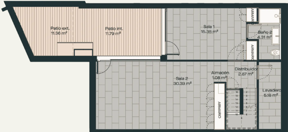
Planta Sótano / BASEMENT FLOOR
