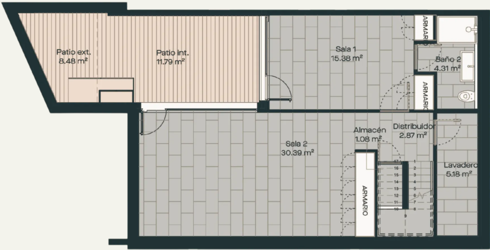
Planta Sótano / BASEMENT FLOOR
