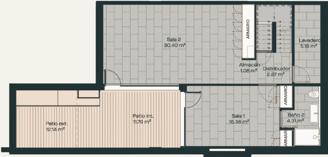
Planta Sótano / BASEMENT FLOOR
